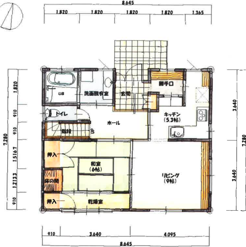
1階平面図
